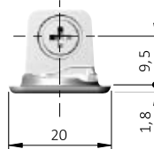
底座附5mm釘套 (18-19mm板厚用)
